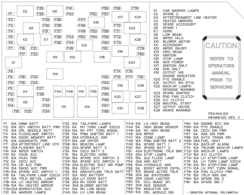
Boîtier de distribution
