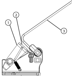
Capot ouvert avec verrou engagé
