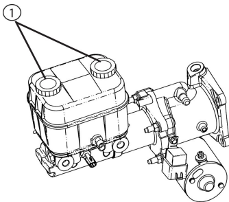
Servo hydraulique de freinage et maître-cylindre
