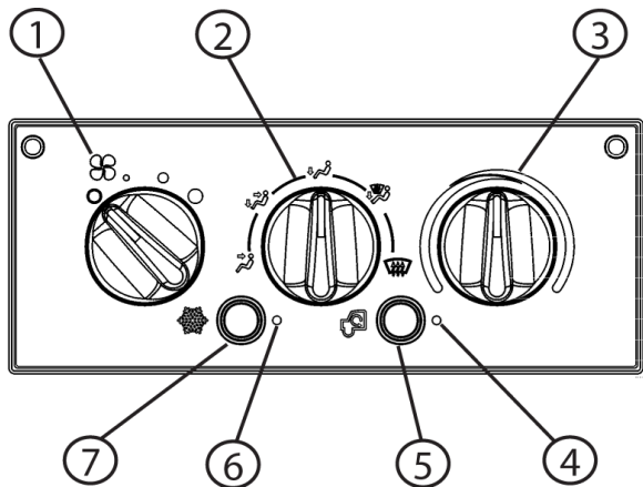
Commandes de chauffage et de climatisation de la cabine
