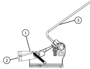
Capot ouvert avec verrou dégage prêt à se fermer
