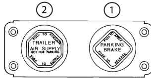
Soupapes de commande des freins de stationnement, combinaison véhicule-remorque
